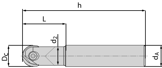
Schaftfräser zylindrisch Form B Vollhartmetall-Schaft / BE.. & TE.. End milling cutter cylindrical form B solid carbide shank / BE.. & TE..
