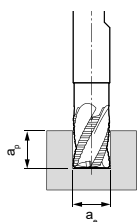
Nutfräsen Groove milling
