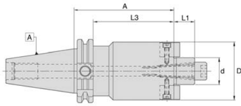
Aufnahme SK40 für Aufsteckfräser Chuck SK40 for face milling cutter
