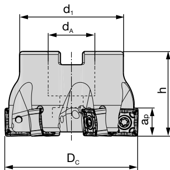
Aufsteckfräser 88° / SN.. 12 Face milling cutter 88° / SN.. 12
